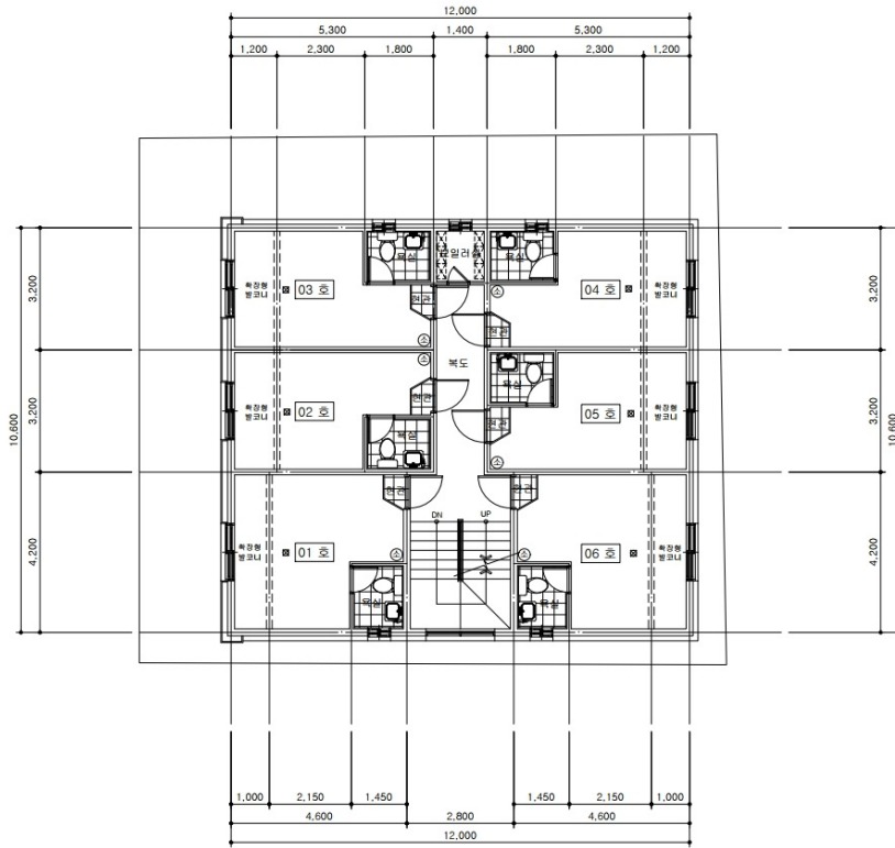
2~3 층 평면도 축척 : 1 / 100
