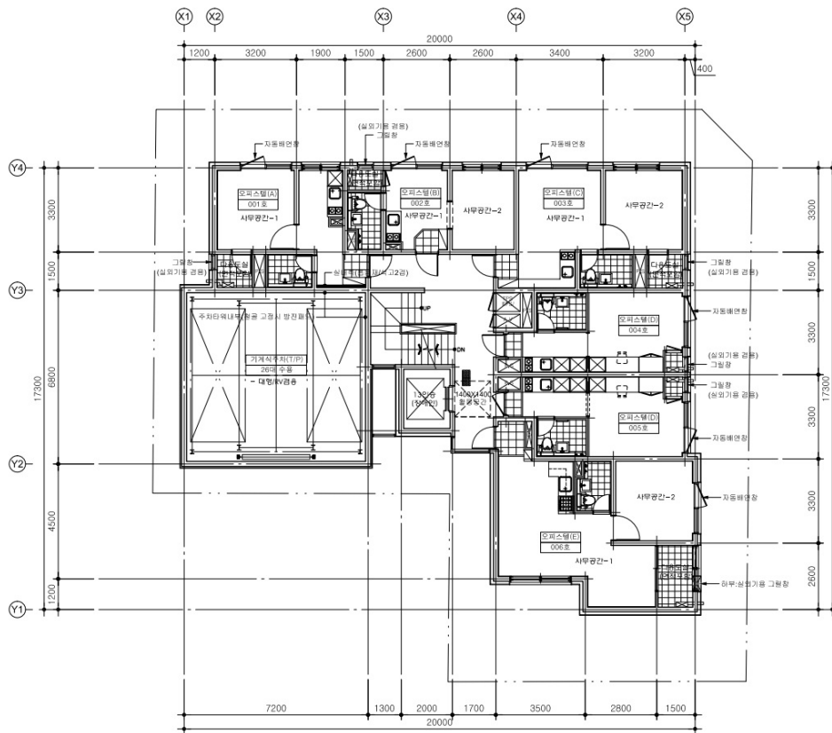
3층 ~ 5층 평면도 SCALE A3 : 1/120
