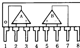
NJM3414AL
