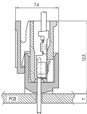
PCB ASS'Y
