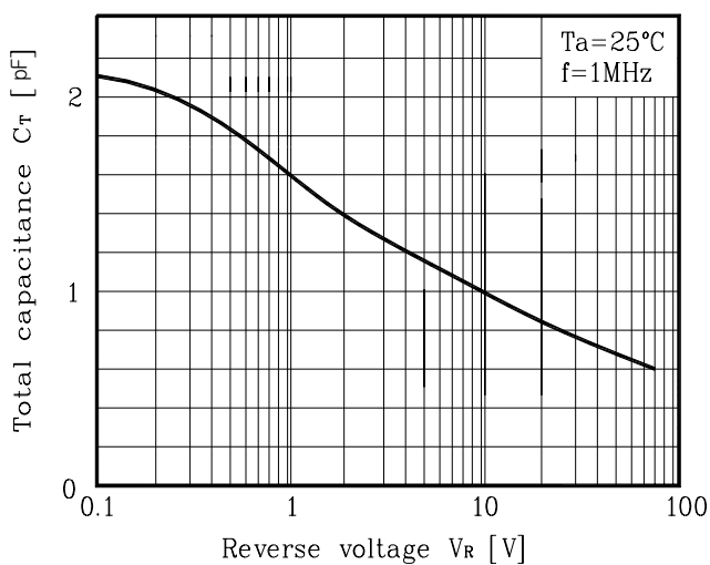
Fig. 3 C_T - V_R
