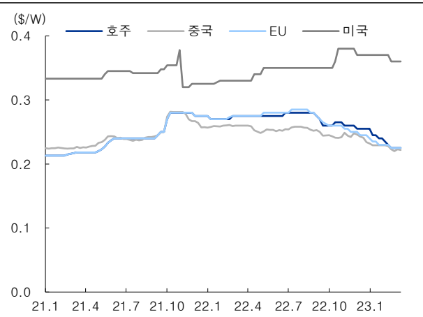
그림 3. 지역별 태양광 모듈 가격 추이
