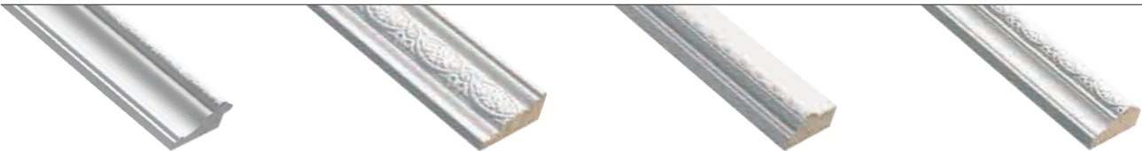
액자몰딩 MG-01 2,400×40×19 포인트몰딩 MG-01 2,400×60×22 포인트몰딩 MG-02 2,400×48×25 포인트몰딩 MG-03 2,400×41×18
